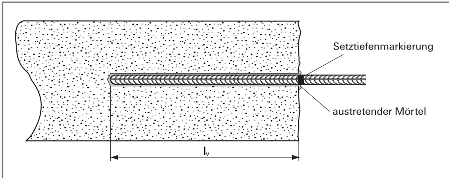
Abb. 11: Setzkontrolle
