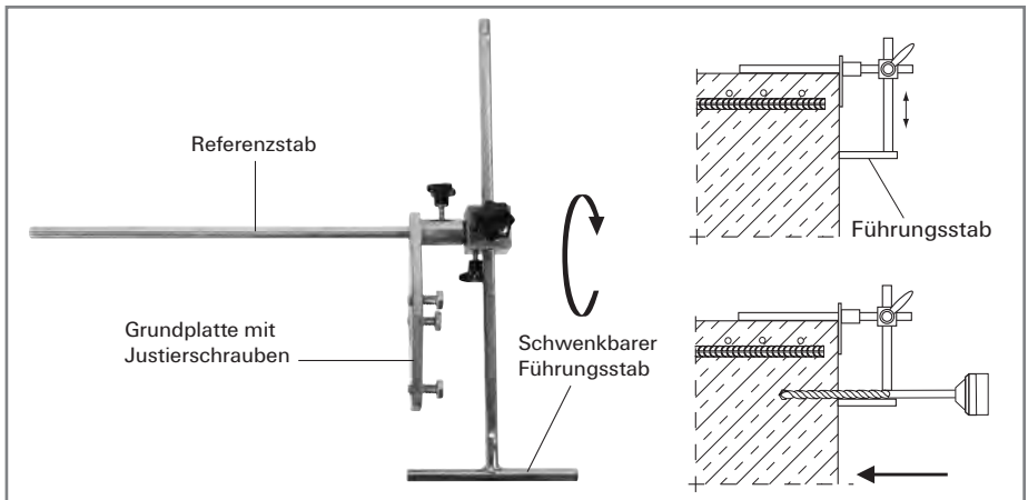
Abb. 6: Bohrhilfe (Grundplatte, Referenzstab, Führungsstab)
